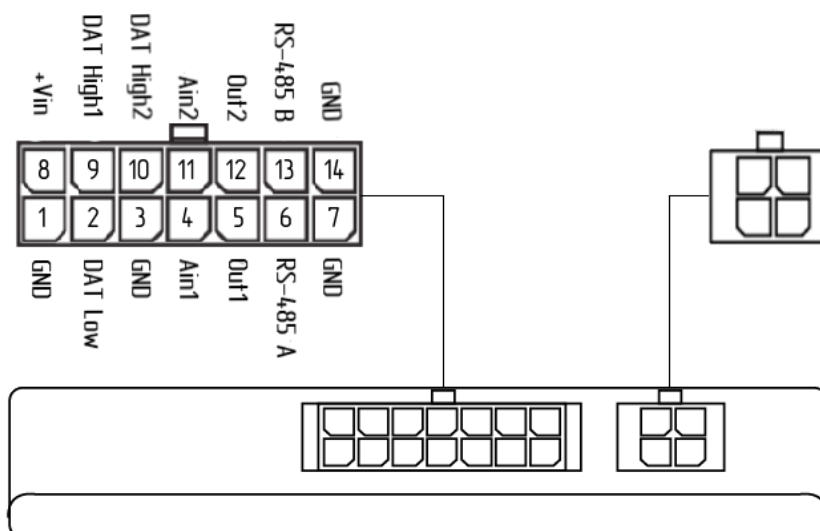
Рисунок 3 – Расположение разъёмов и нумерация контактов.
