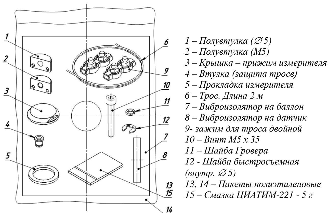
Рис 5.2 – Состав комплекта фиксации измерителя
