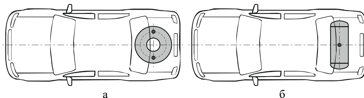
Рис. 2.1 – Типичное расположение топливных баллонов ГБО и рекомендованные места установки измерителя датчика в легковых автомобилях (а – торoidalный баллон, б – цилиндрический баллон)
